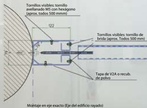
Guías laterales
